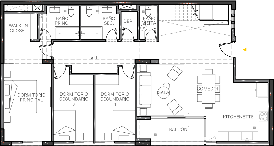
NIVEL SUPERIOR
