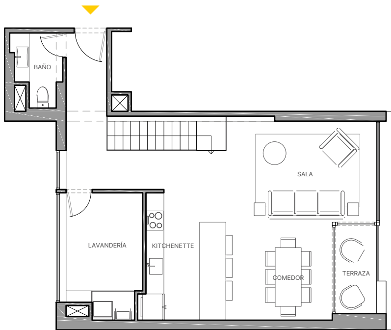
NIVEL 1
